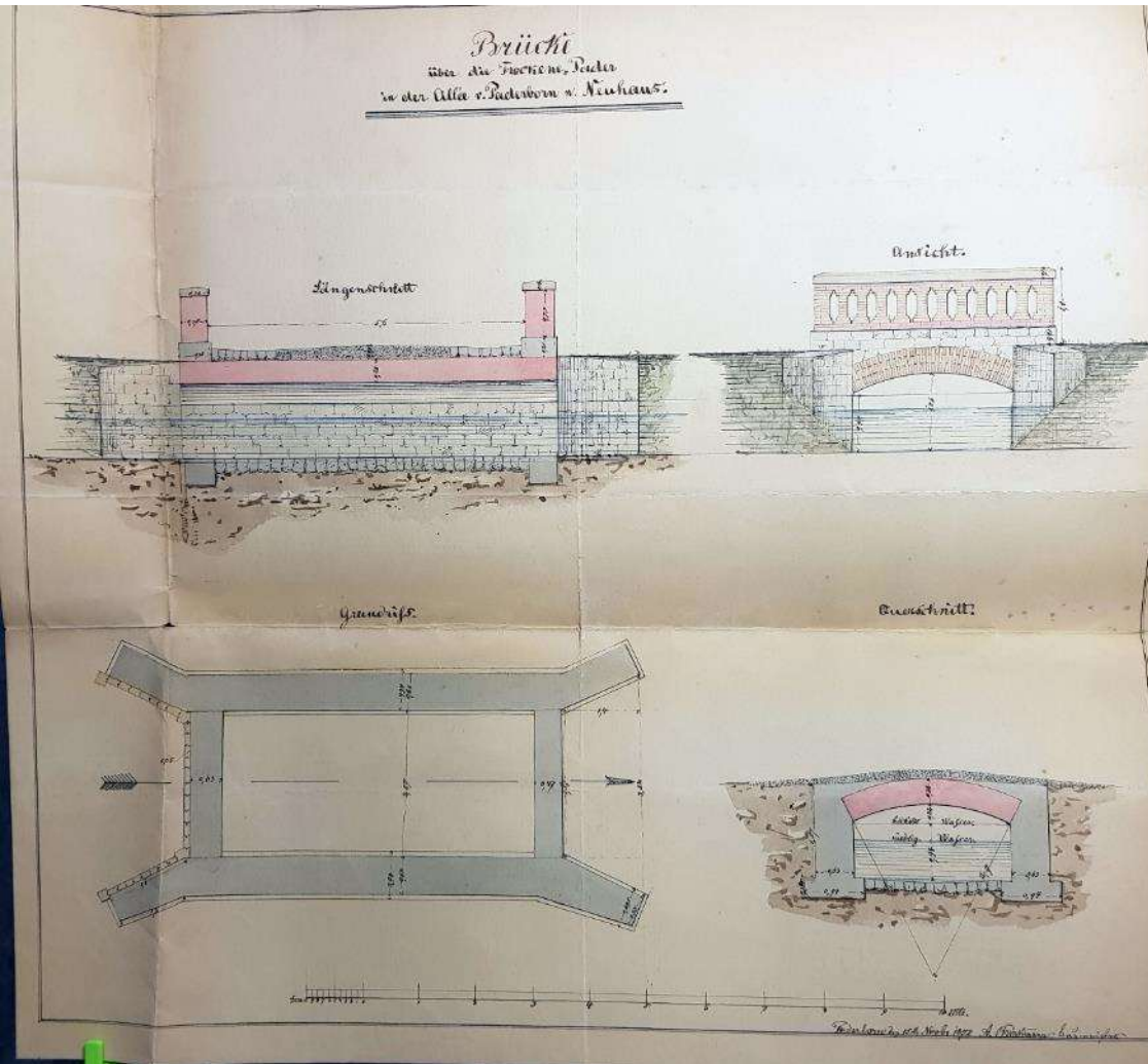
Modernisierung der Holzbrücke, Entwurf 1872 (StadtA Pb, A 716, unfol.)
