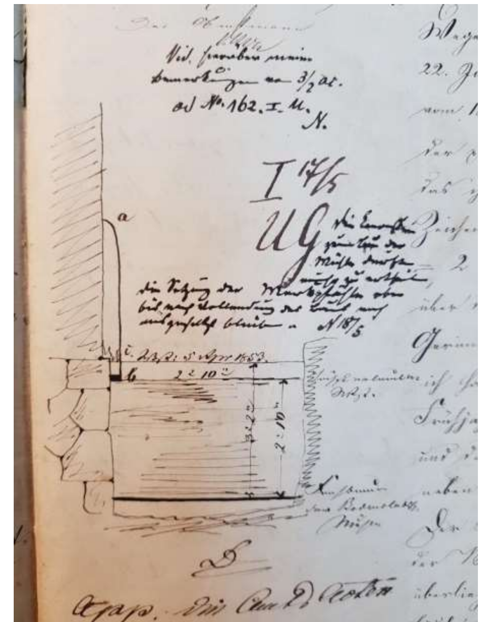
Handskizze Stauwerk mit „Merkpfahl“, 1853 (LA Detmold, Reg. Minden, I U Nr. 660, unfol.)
